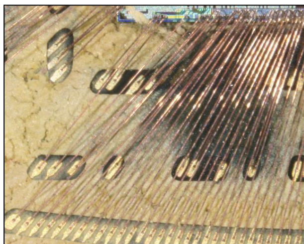
Cuワイヤ全体像
