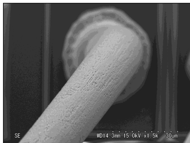
1st側: Cuワイヤ腐食なし
