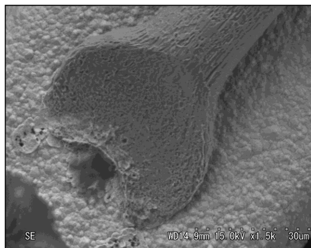
2nd側: Cuワイヤ腐食なし
